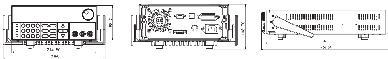
IT6723H/IT6724H/T6723G 機型尺寸圖
