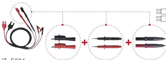
IT-E604 黑色直插插頭-通用表筆+鱷魚夾
