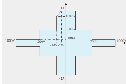
IT2801 1000V輸出特性曲線
