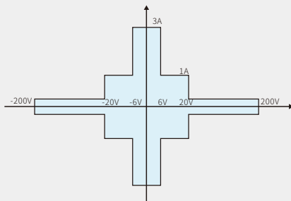
IT2806 200V輸出特性曲線 (直流或脈衝)
