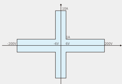
IT2806 200V輸出特性曲線 (僅脈衝)
