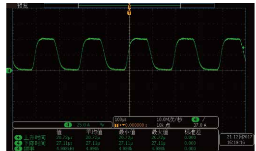
IT8906A-1200-240 5kHz動態拉載0A-50A
