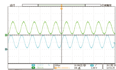
10kHz正弦波
