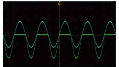
负半波整流
