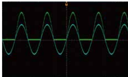
正半波整流
